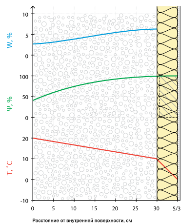
в1 – мокрое утепление по минвате 50 мм
