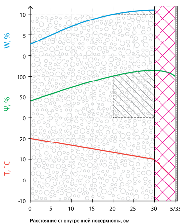
б1 – мокрое утепление по ППС 50 мм
