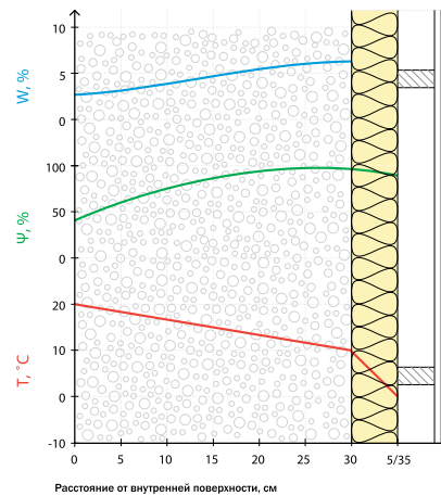
г1 – минвата и облицовка на отnose
