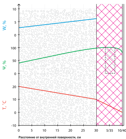
б2 – мокрое утепление по ППС 100 мм
