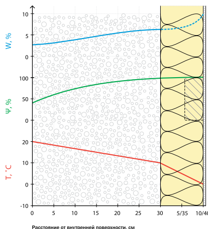
в2 – мокрое утепление по минвате 100 мм
