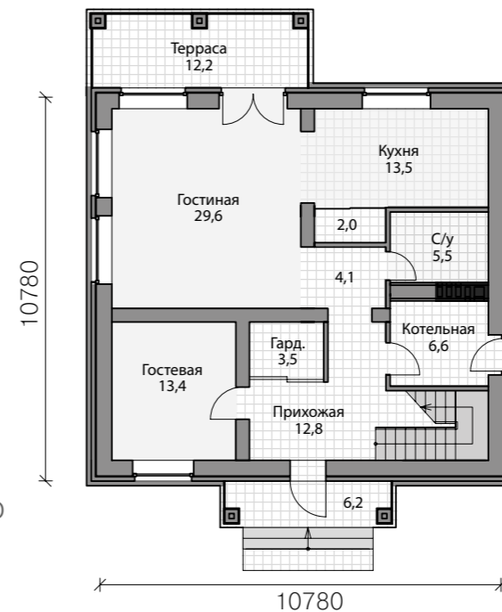
ПЛАН ПЕРВОГО ЭТАЖА
