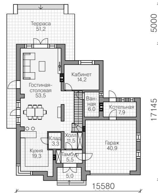
ПЛАН ПЕРВОГО ЭТАЖА
