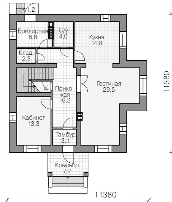
ПЛАН ПЕРВОГО ЭТАЖА
