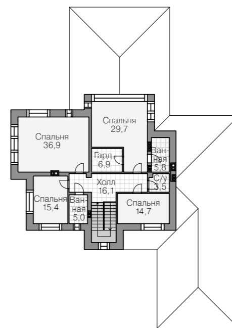
ПЛАН ВТОРОГО ЭТАЖА
