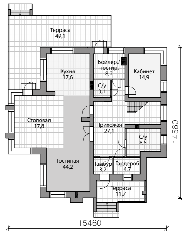
ПЛАН ПЕРВОГО ЭТАЖА
