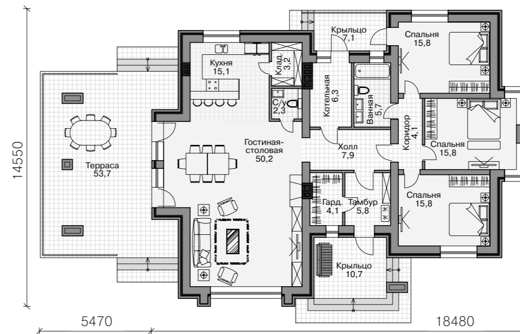
ПЛАН ПЕРВОГО ЭТАЖА
