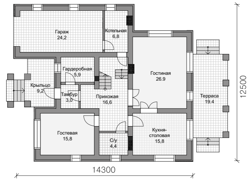
ПЛАН ПЕРВОГО ЭТАЖА
