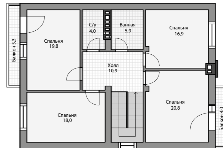
ПЛАН ВТОРОГО ЭТАЖА
